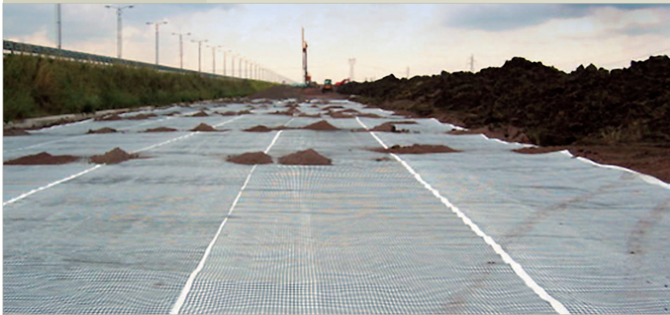
Il geocomposito TENAX GT 330
